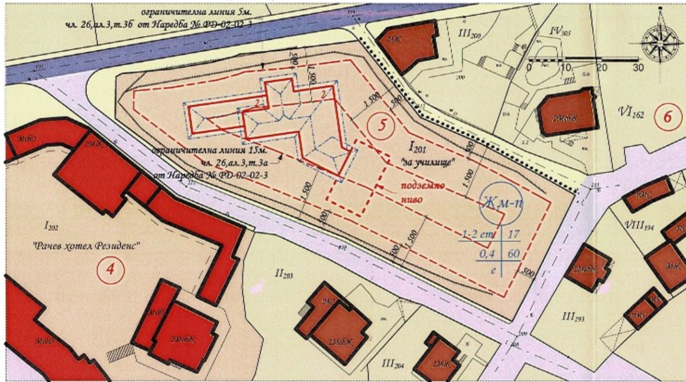
ЧМ на ПУП - план за застрояване за УПИ I-201, кв. 5 по плана на село Арбанаси, Община Велико Търново, Област Велико Търново, М 1:1000
