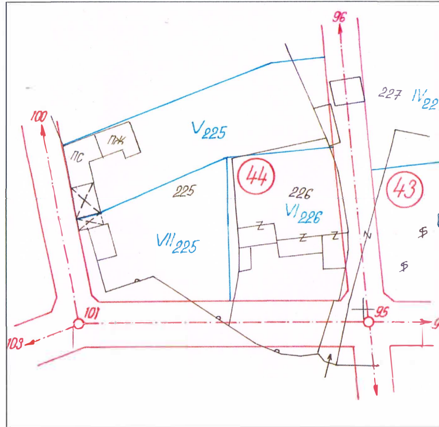
ЧИ НА ПУП - ПЛАН ЗА РЕГУЛАЦИЯ М 1:1 000
