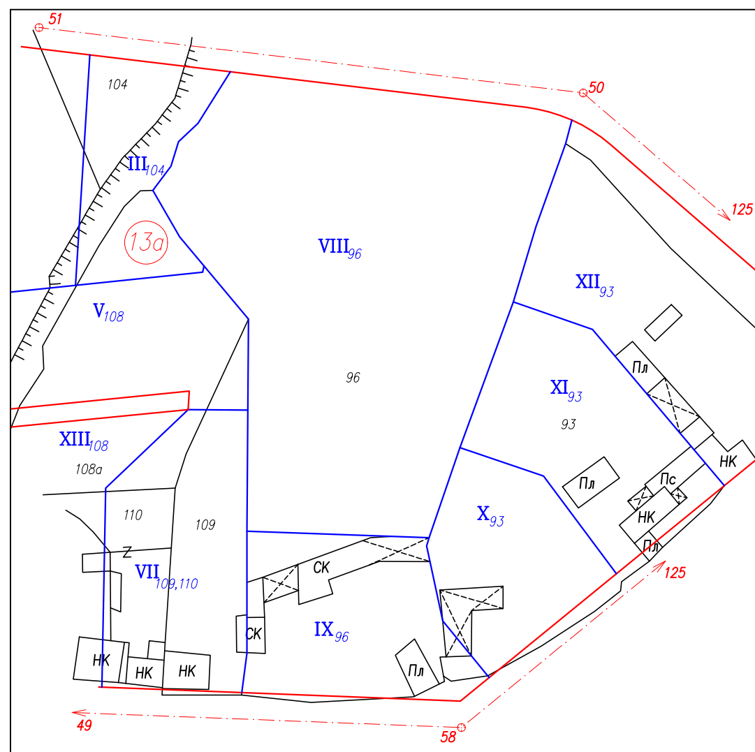
ИЗВАДКА ОТ ПЛАНА ЗА РЕГУЛАЦИЯ М 1:1 000
