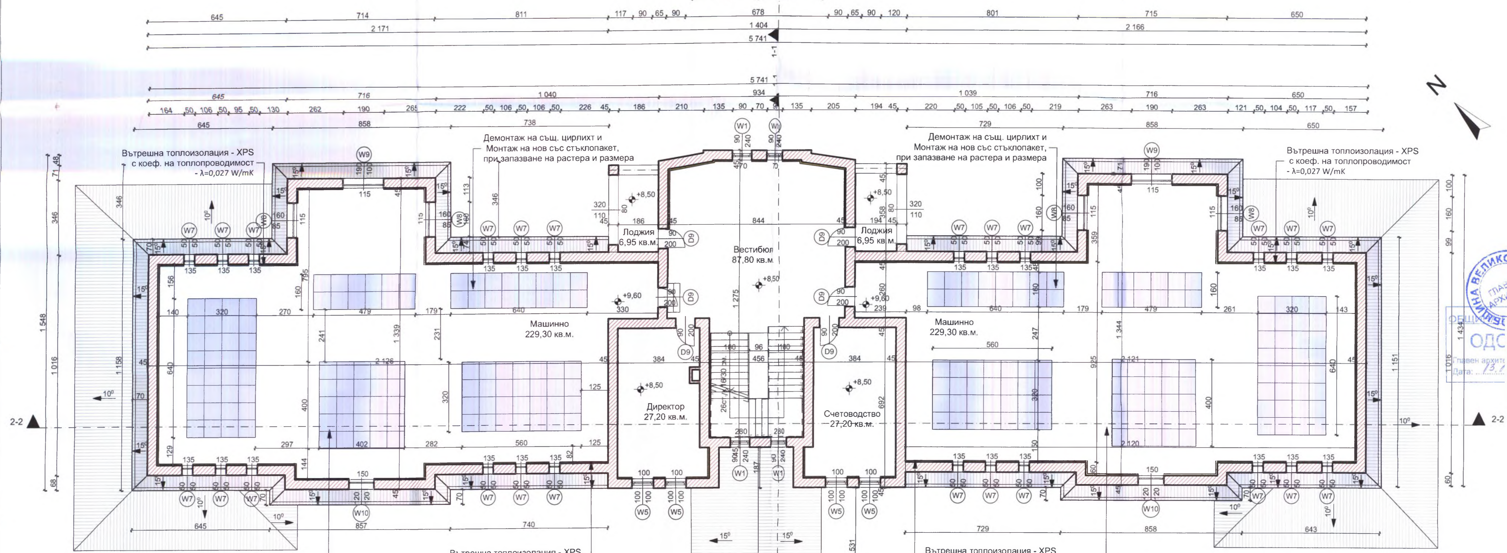
РАЗПРЕДЕЛЕНИЕ НА КОТА +8,50 м. М 1:100
