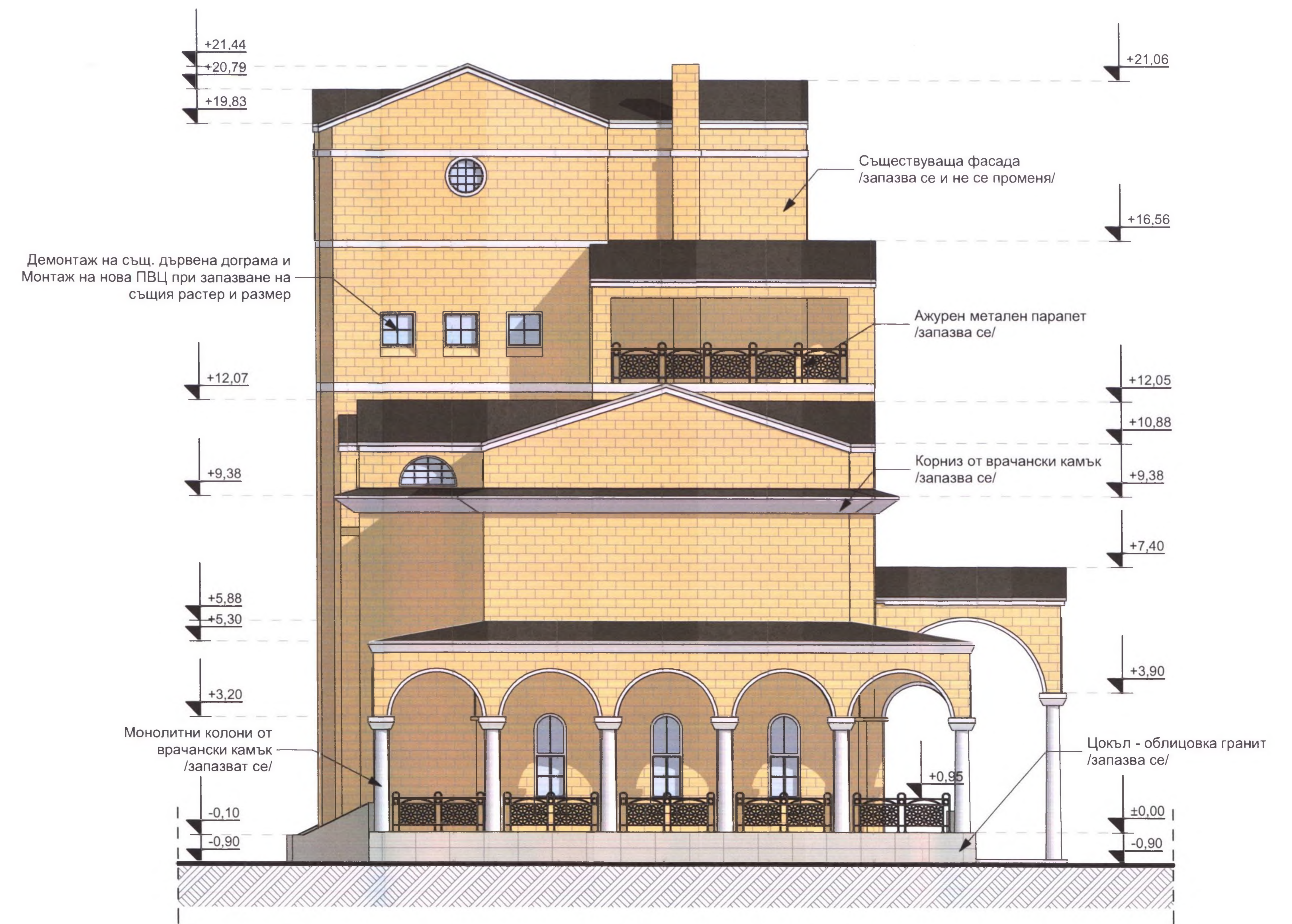
ФАСАДА "СЕВЕРОЗАПАД" М 1:100
